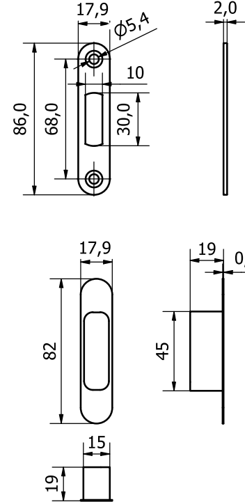
protiplech + vanička
