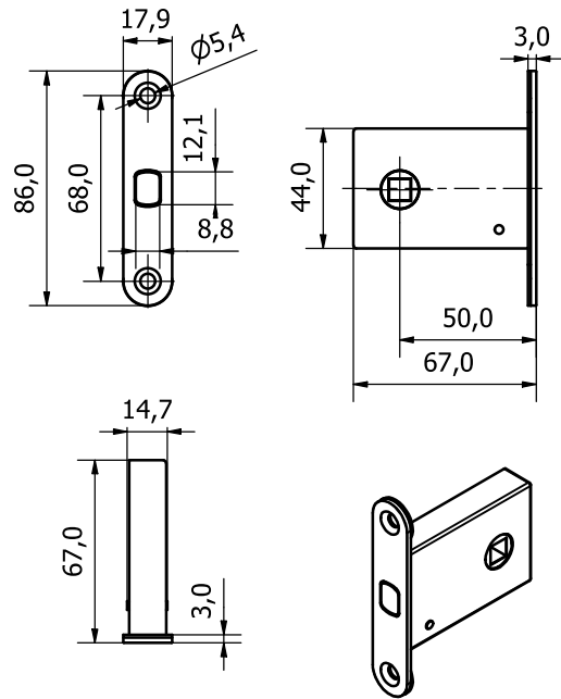
frézování dveří
