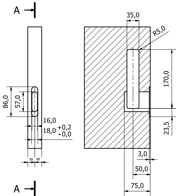
frézování dveří
